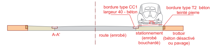
Profil avec stationnement longitudinal
