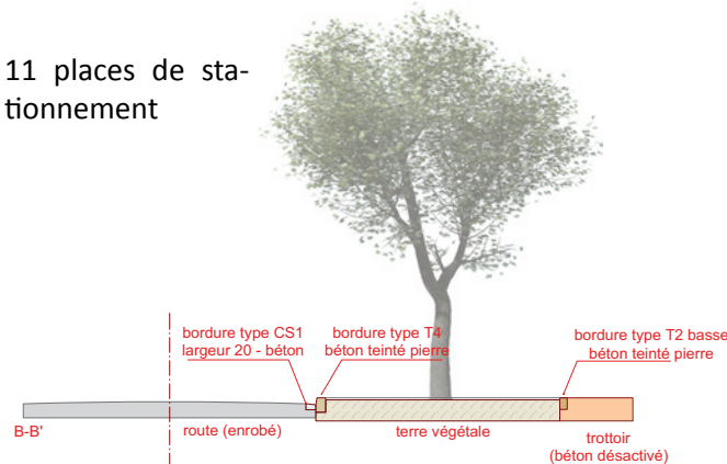
Profil avec stationnement en bataille
