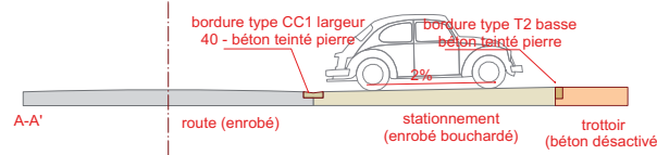
Profil avec stationnement en bataille
