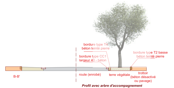
Profil avec arbre d'accompagnement
